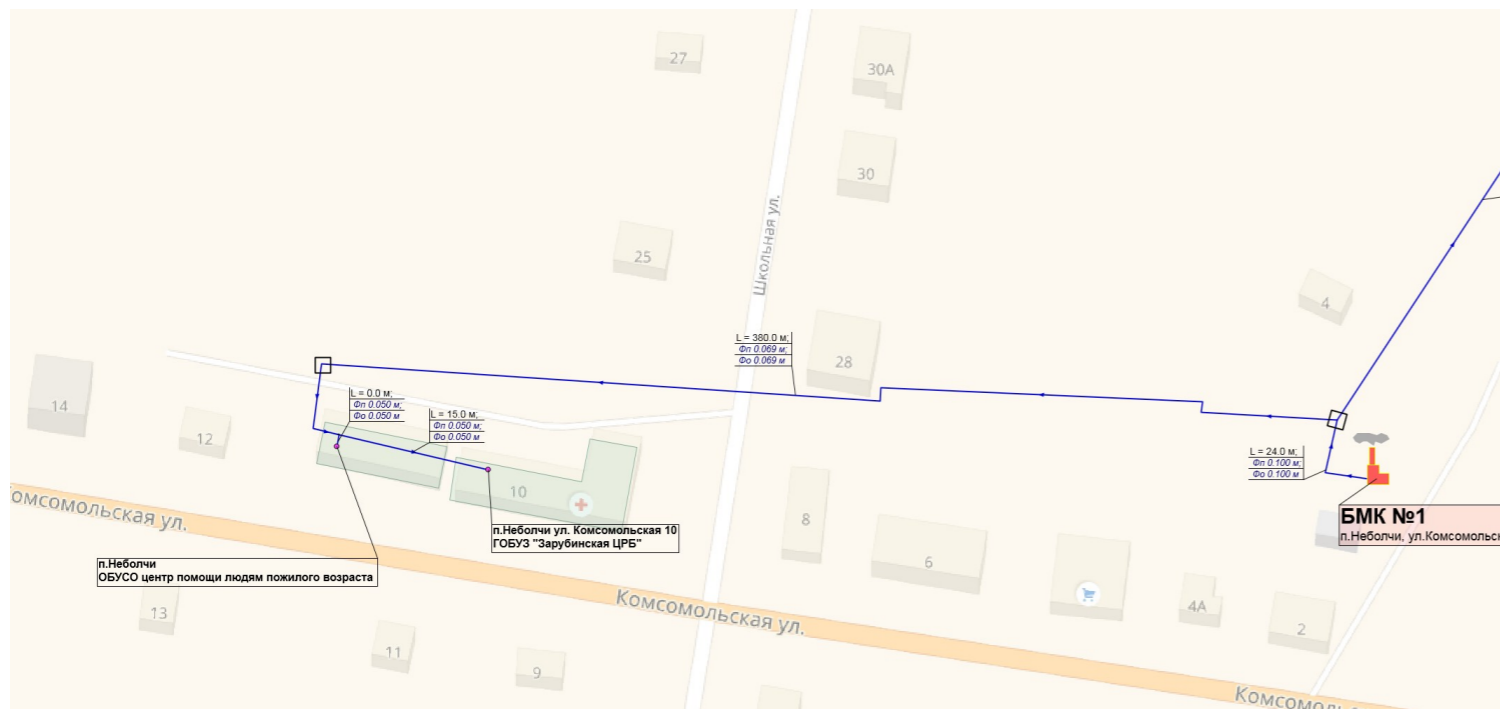
Рисунок 1.1 Схема тепловых сетей котельной БМК №1 п. Неболчи, ул. Комсомольская
